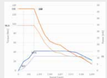
Diagramma Potenza / Coppia del Mandrino
