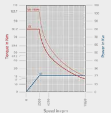
Diagramma Potenza / Coppia Mandrino ad Alta Velocità
